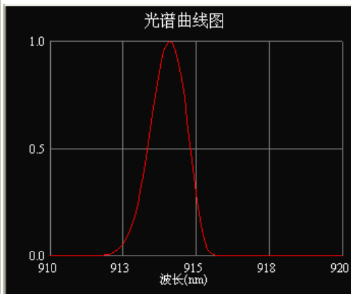
光谱曲线
