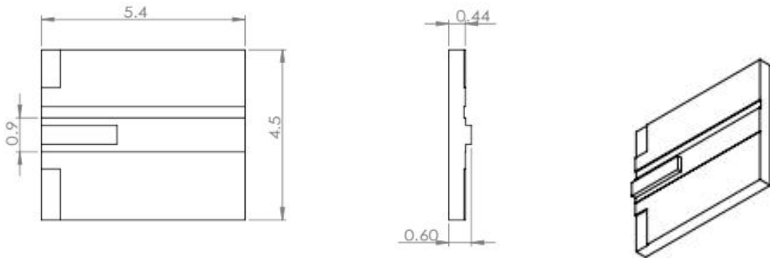
CoS 封装
