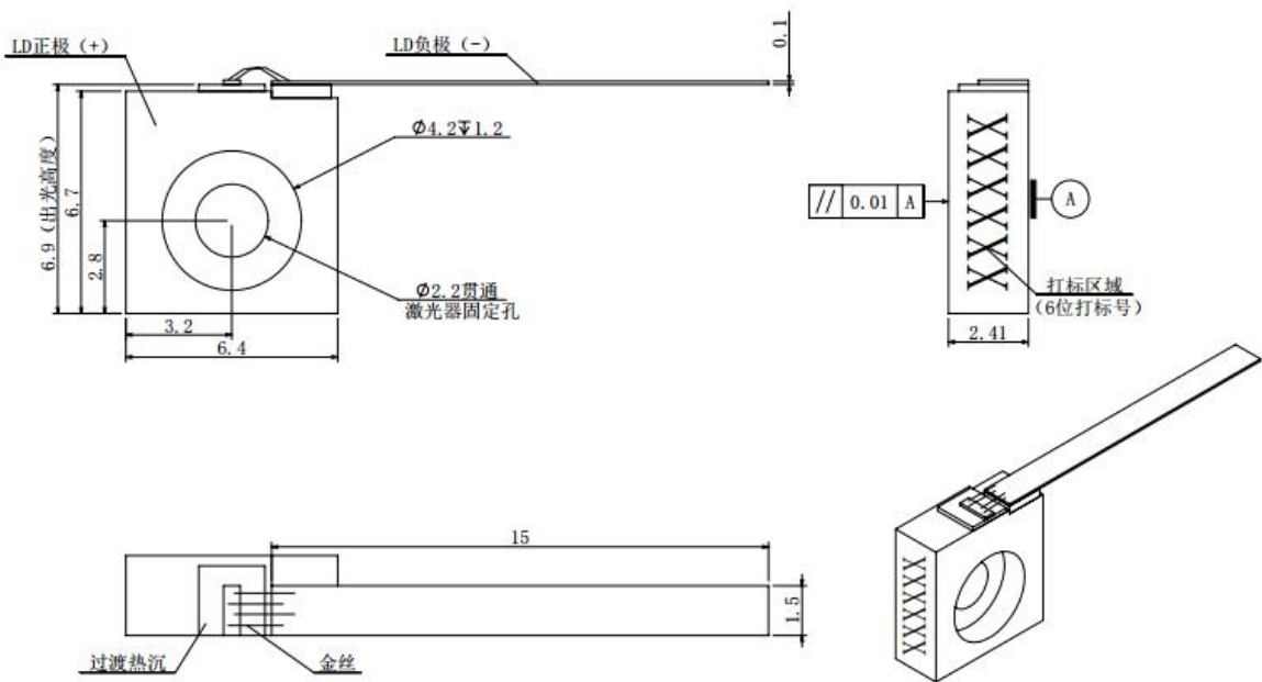
C 封装
