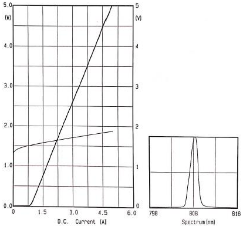
P-I-V 曲线
